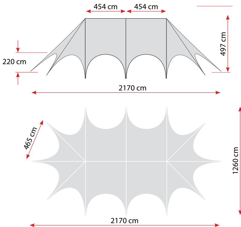
Rys. 1. Przekrój pionowy i rzut poziomy namiotu JEHLAN
