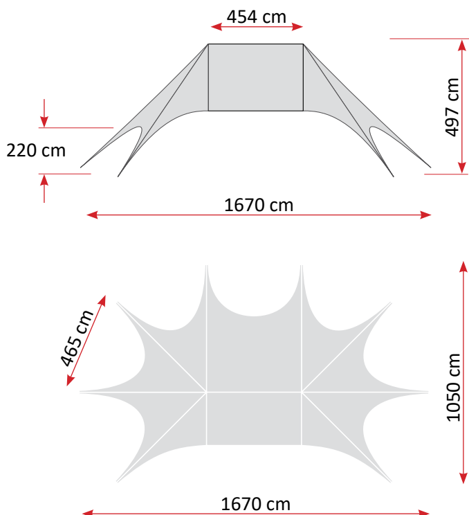
Rys. 1. Przekrój pionowy i rzut poziomy namiotu JEHLAN
