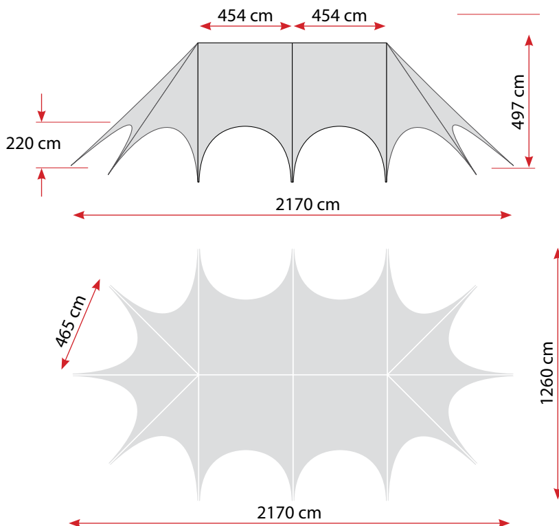
Obr. 1: bokorys a půdorys stanu
