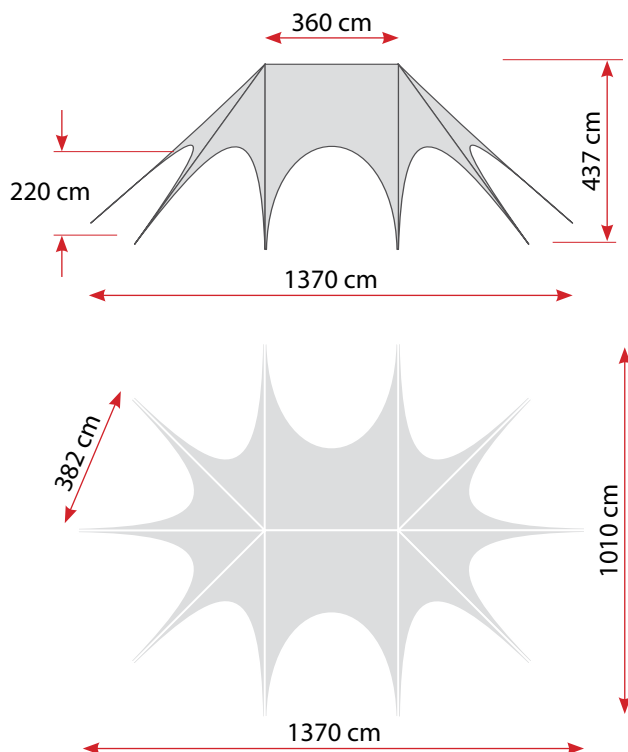
Obr. 1: bokorys a půdorys stanu
